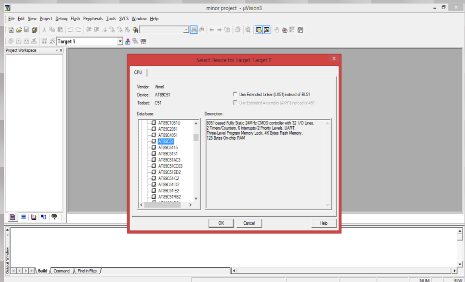
Fig. 5: Kiel Uvision 3
